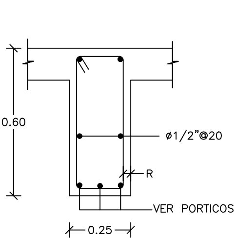
10 SECCION "P1" ES-08 ESC. 1:15
