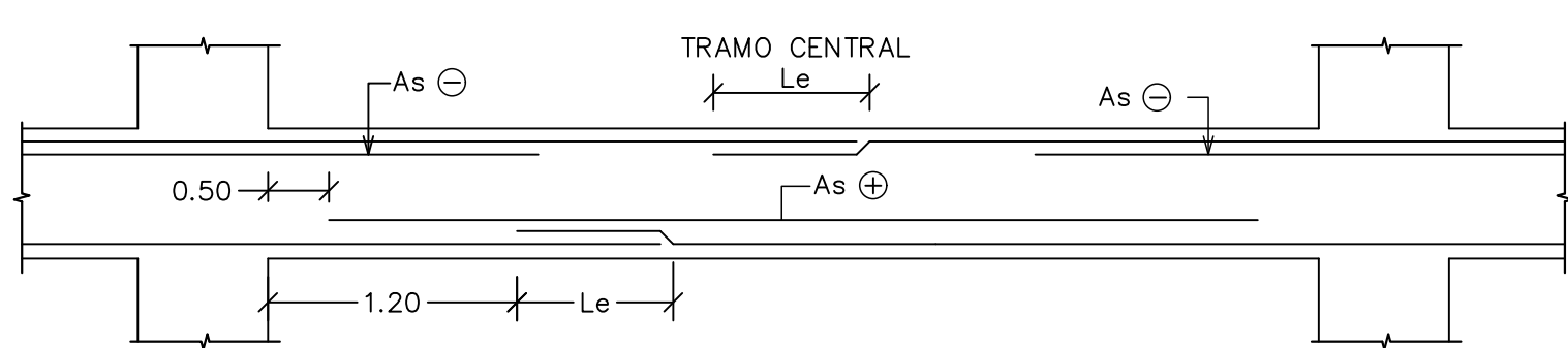
4 DETALLE DE EMPALME ES-08 ESC. 1:75
