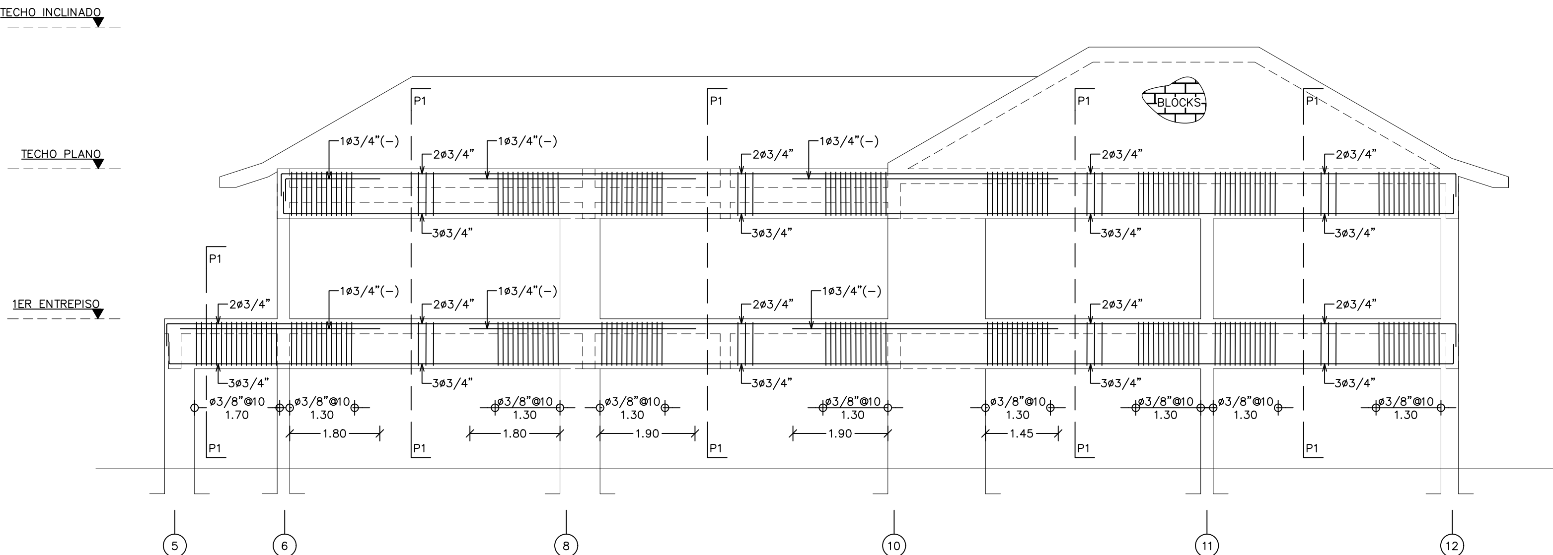
2 DETALLE PORTICO "CX" ES-08 ESC. 1:75
