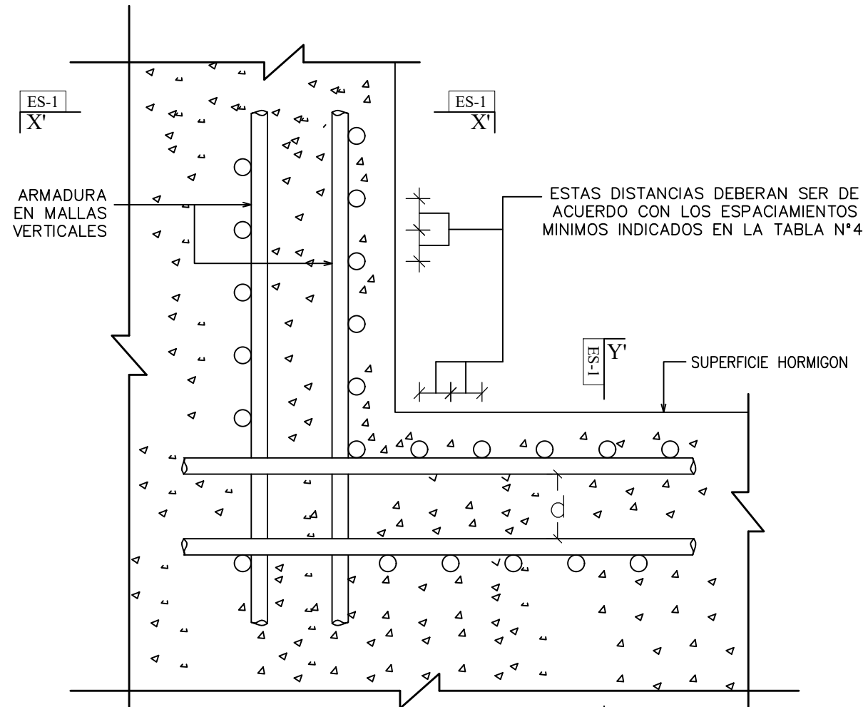
16 SECCION X'-X'
