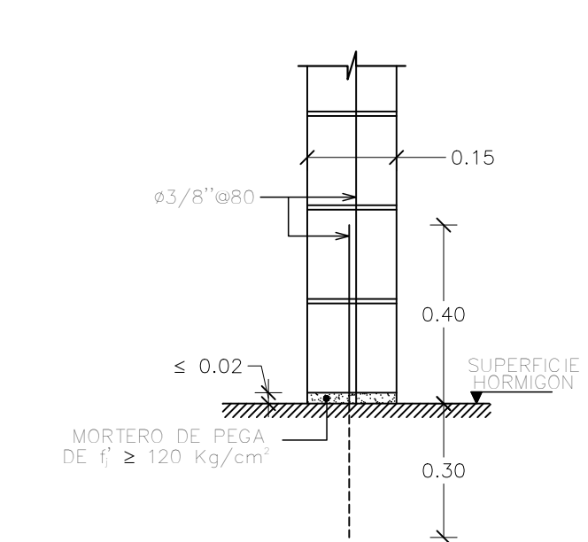
7 SECCION "d-d" ES-08 ESC. S/E
