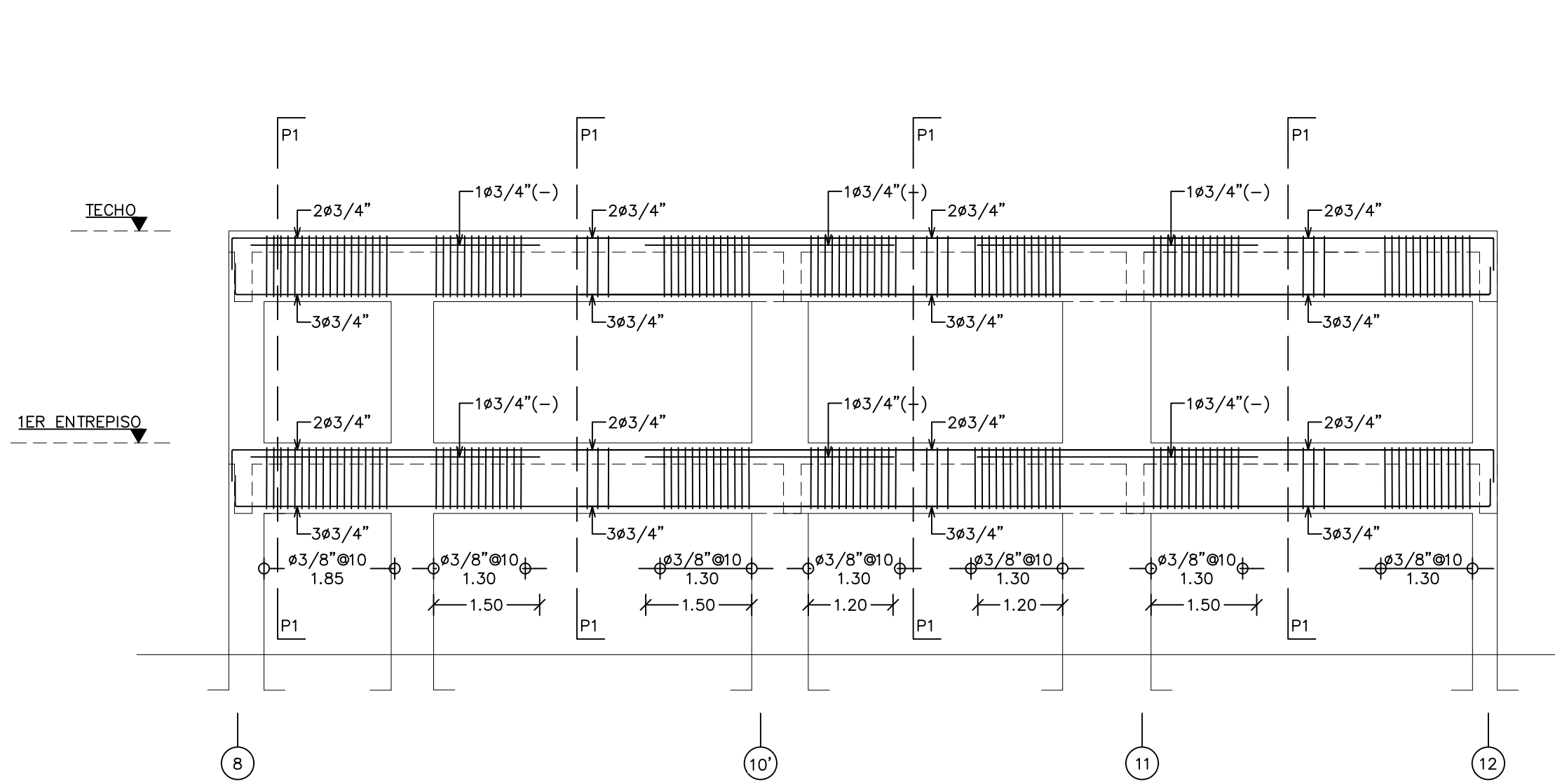
1 DETALLE PORTICO "AX" ES-08 ESC. 1:75
