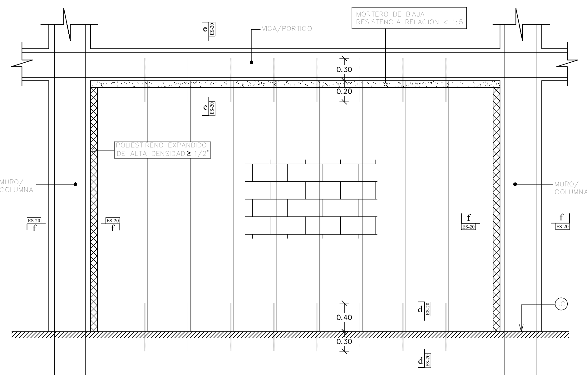
3 DETALLE UNION PORTICO MAMPOSTERIA ES-08 ESC. 1:75
