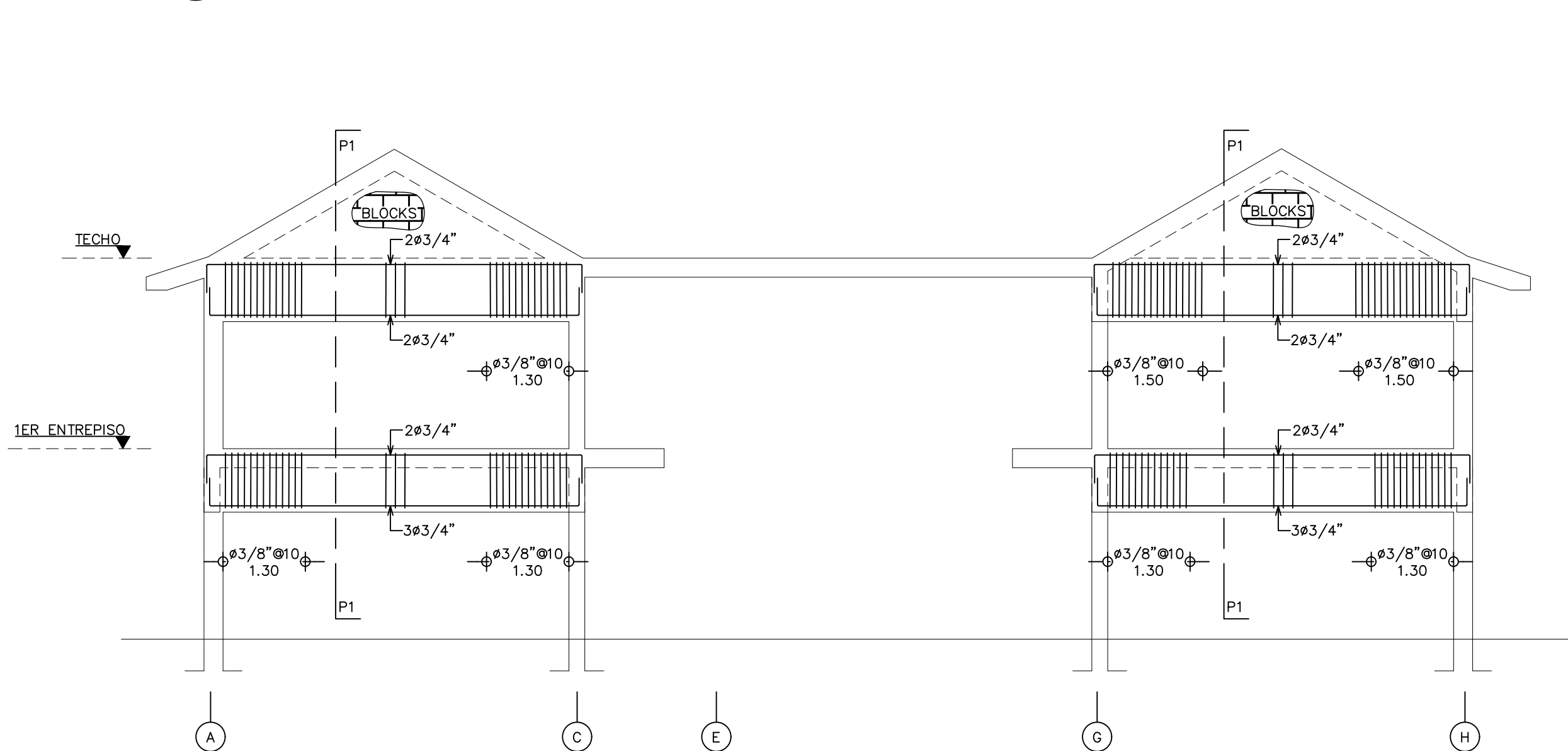
8 DETALLE PORTICO "10' Y" ES-10 ESC. 1:75
