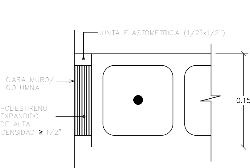
9 SECCION "f-f" ES-08 ESC. S/E
