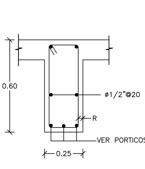
7 SECCION "P4" ES-10 ESC. 1:15
